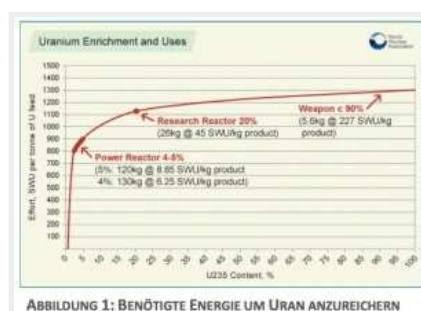
ABBILDUNG 1: BENÖTIGTE ENERGIE UM URAN ANZUREICHERN
